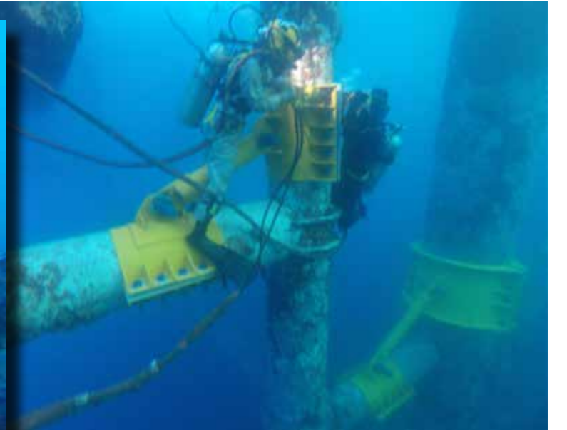
جزئیاتی نزدیک‌تر از عملیات تقویت سازه پهلوگیری سکو PLQ میدان بلال
